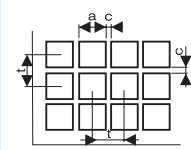
Štvorcové otvory radové
