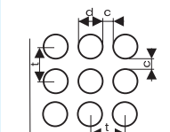
Kruhové otvory radové
